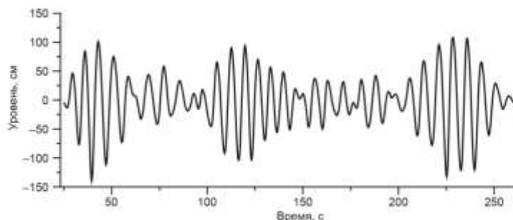
Рис. 3.17. Пример развитой групповой структуры волны во время шторма (23.12.2008 г., МЛСП D-6)
