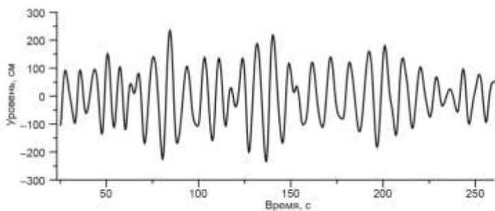
Рис. 3.18. Пример неоднородной структуры волны (21.12.2008 г., МЛСП D-6)
