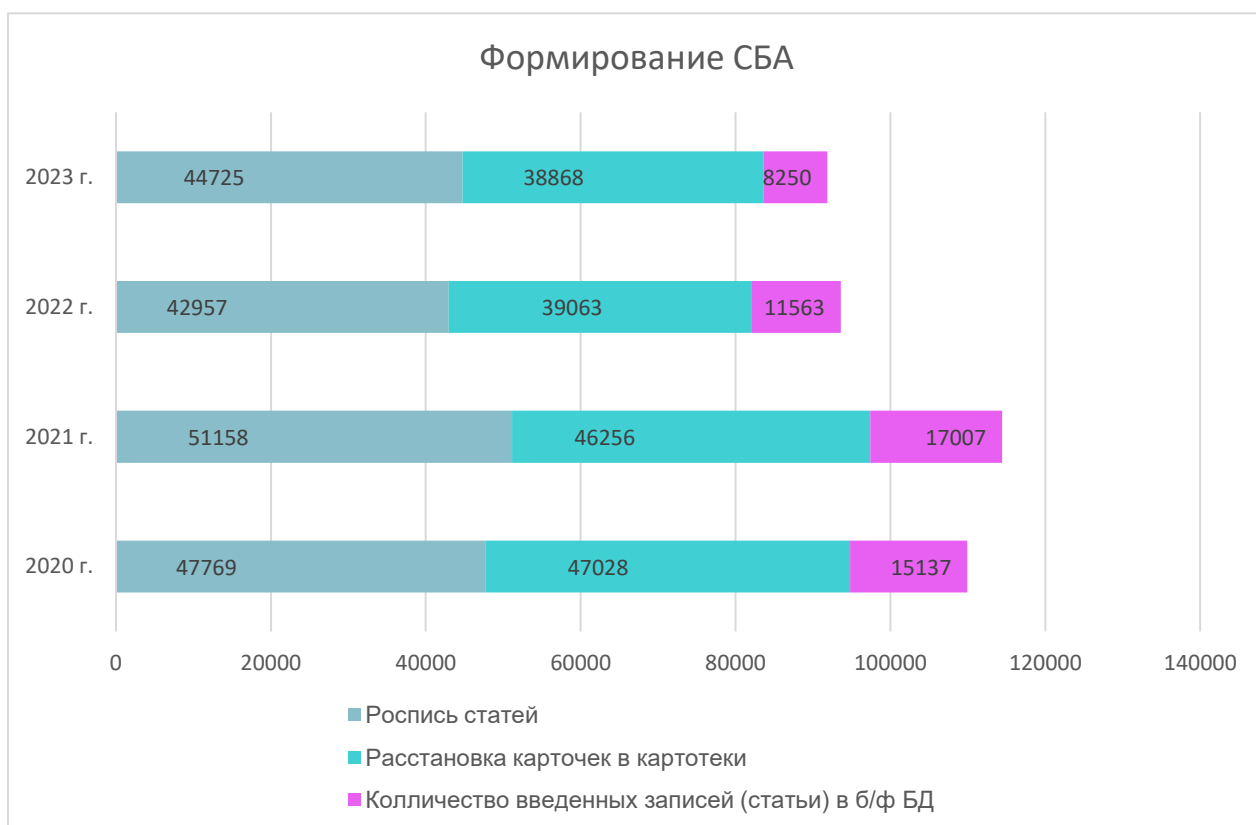
Рис. 1. Формирование СБА
