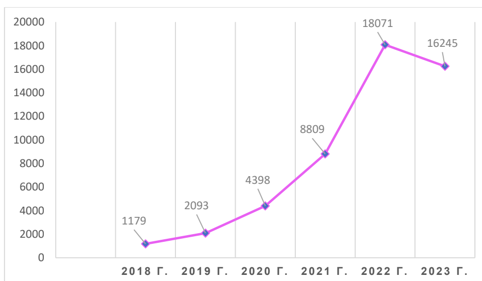
Рис. 6. Виртуальные справки
